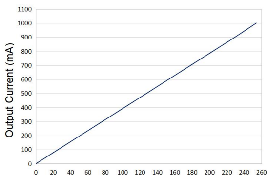
Linear dimming
